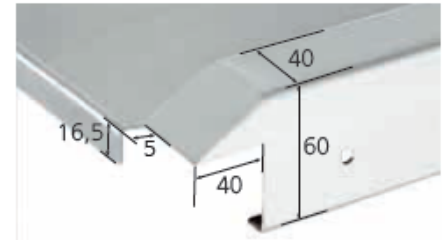
Standard-Befestigungsprofil
