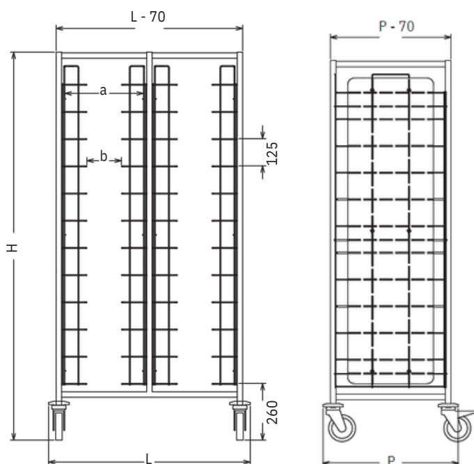
Wagen 2 x 12 Ebenen, breiter Einschub (doppelte Einschubseite nebeneinander). Vorderansicht.
