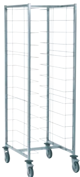
2x12 Ebenen mit doppeltem Einschub (Rücken an Rücken) in Längsrichtung.
